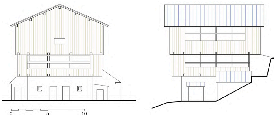
Fienile con ballatoio Prospetto del fronte rivolto a valle e prospetto laterale
